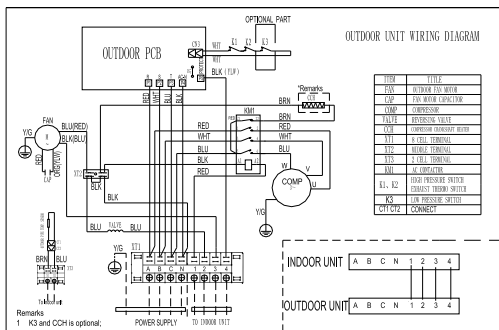
Схема для наружных блоков (Модель LAC-36T)
