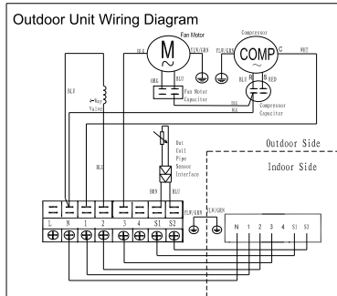
Схема для наружных блоков (Модель LAC-18T)
