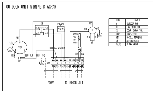
Схема для наружных блоков (Модель LAC-24T)
