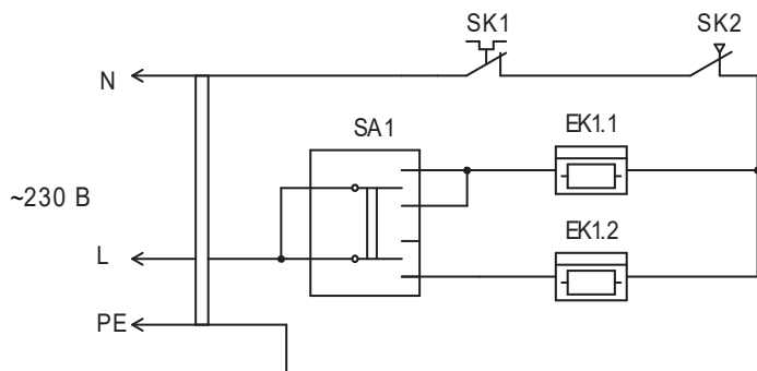
Рис. 9 Схема электрическая принципиальная конвекторов ВНСI-1000 SM со стич элементом без датчика опрокидывания
