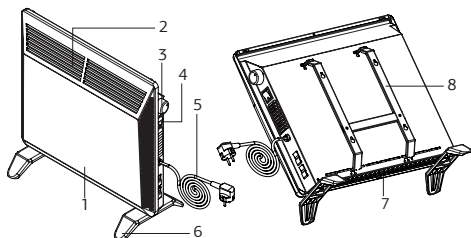
Рис. 2 Устройство конвектора (изображение может отличаться в зависимости от марки конвектора)
