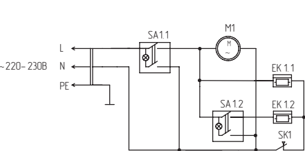
Схема электрическая модель LTZ-3.0 S
